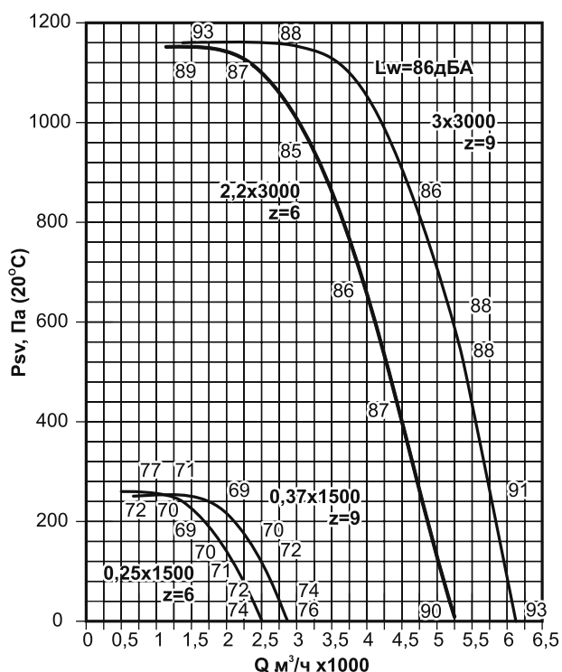
Рис. 144. Аэродинамическая характеристика вентилятора ВКРВм №3,55.
