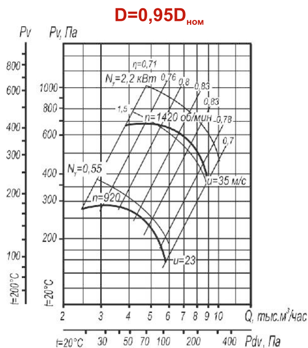
Рис. 53. Аэродинамическая характеристика вентилятора BP 80-75 №5 исп-1; 5 D=0,95D_{\text{НОМ}} .
