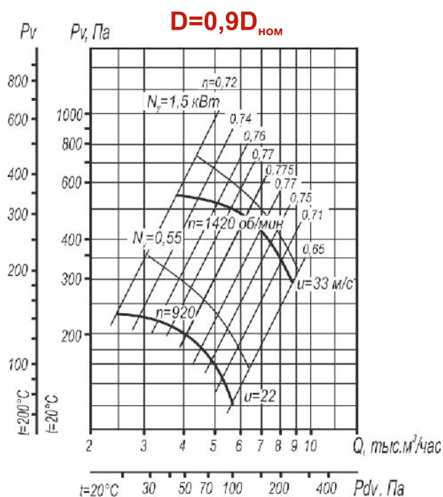
Рис. 52. Аэродинамическая характеристика вентилятора BP 80-75 №5 исп-1; 5 D=0,9D_{\text{НОМ}} .
