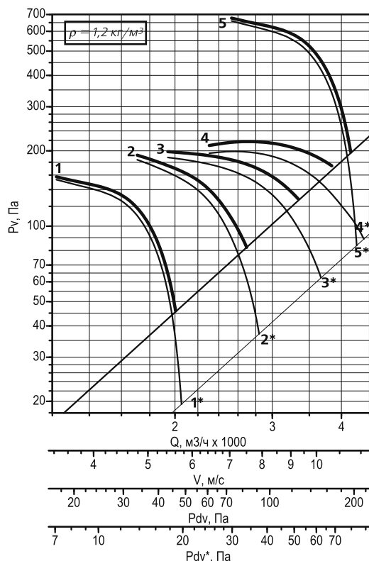
Рис. 262. Аэродинамическая характеристика осевого вентилятора дымоудаления ВОДм-ДУ №4.
