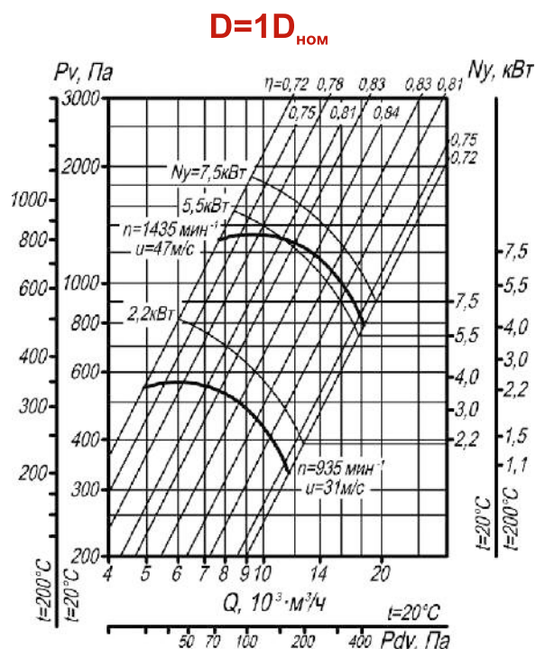
Рис. 56. Аэродинамическая характеристика вентилятора ВР 80-75 №6,3 исп-1; 5 D=1D_{\text{НОМ}} .
