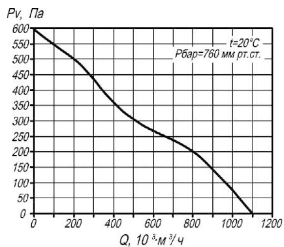
Рис. 199. Аэродинамическая характеристика вентилятора канального КВКр 250.
