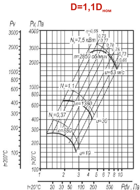
Рис. 50. Аэродинамическая характеристика вентилятора ВР 80-75 №4 исп-1, D=1,1D_{\text{ном}} .
