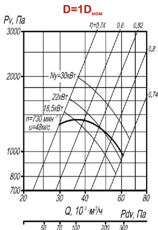
Рис. 68. Аэродинамическая характеристика вентилятора ВР 80-75 №12,5 исп-1 D=1D ном .
