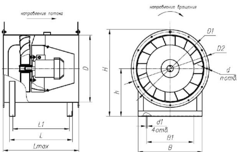
Рис. 179. Габаритные и присоединительные размеры вентиляторов осевых ВО 30-160.
