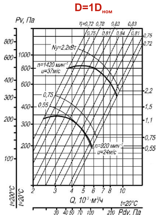
Рис. 51. Аэродинамическая характеристика вентилятора ВР 80-75 №5 исп-1; 5 D=1D_{\text{ном}} .
