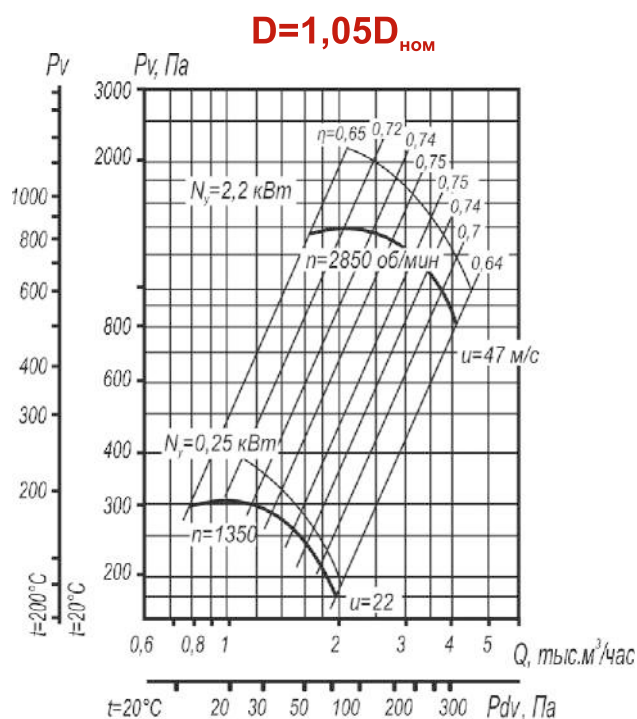
Рис. 44. Аэродинамическая характеристика вентилятора ВР 80-75 №3,15 исп-1, D=1,05D_{\text{НОМ}} .
