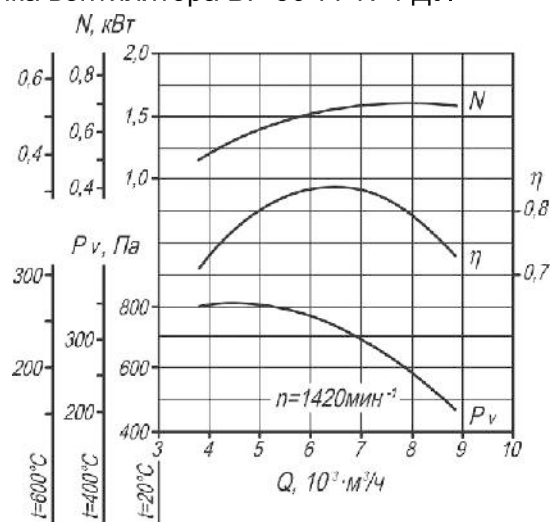
Рис. 217. Аэродинамическая характеристика вентилятора ВР 86-77 №4 ДУ.
