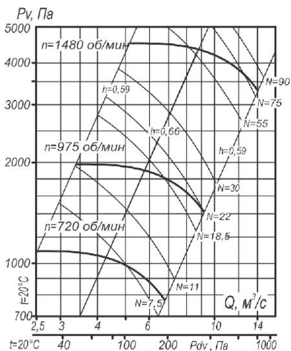
Рис. 117. Аэродинамическая характеристика вентилятора BP №140-40 №10.
