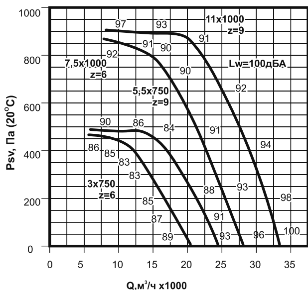
Рис. 152. Аэродинамическая характеристика вентилятора ВКРВм №9.
