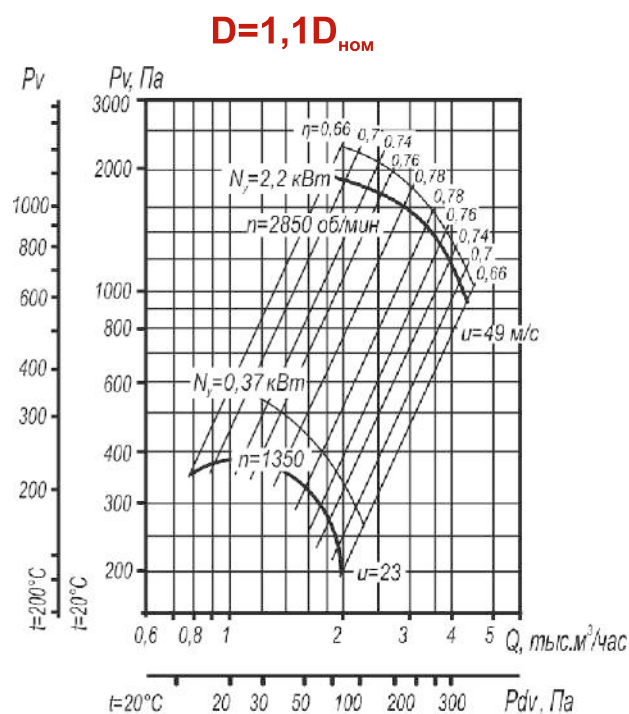
Рис. 45. Аэродинамическая характеристика вентилятора ВР 80-75 №3,15 исп-1, D=1,1D_{\text{НОМ}} .
