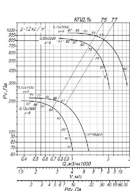
Рис. 75. Аэродинамическая характеристика вентилятора BP 80-75 №2,8 исп-1.
