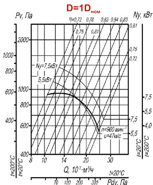
Рис. 61. Аэродинамическая характеристика вентилятора BP 80-75 №8 исп-1; 5 D=1D ном .
