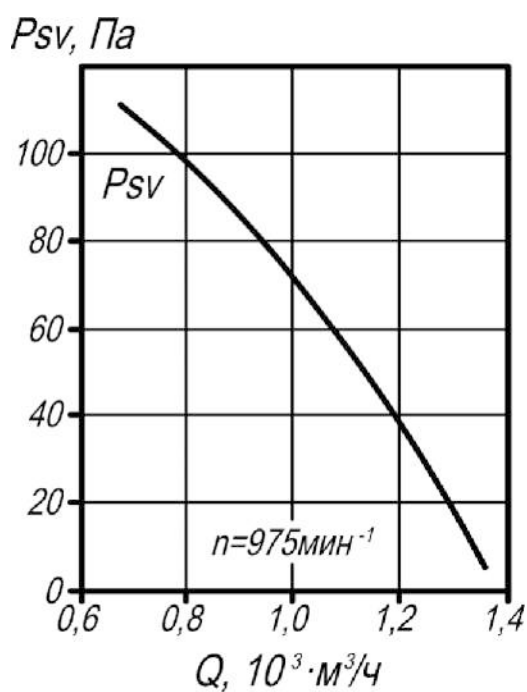
ВКРм-3,15
