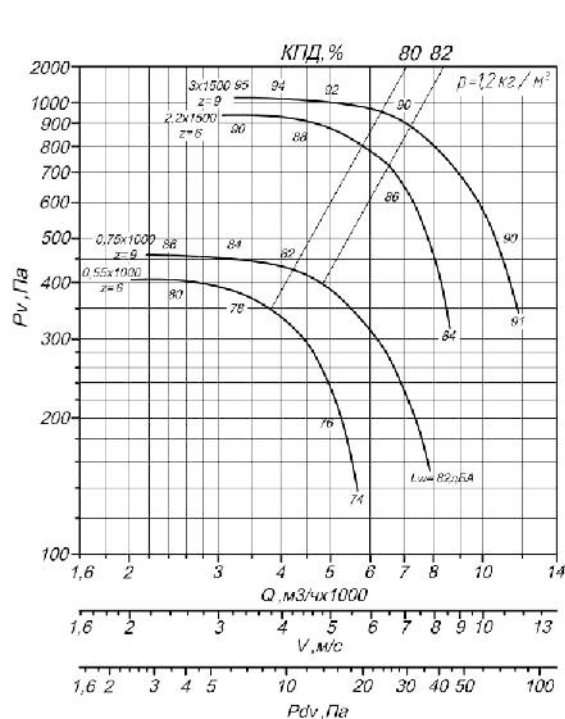
Рис. 78. Аэродинамическая характеристика вентилятора BP 80-75 №5,6 исп-1.
