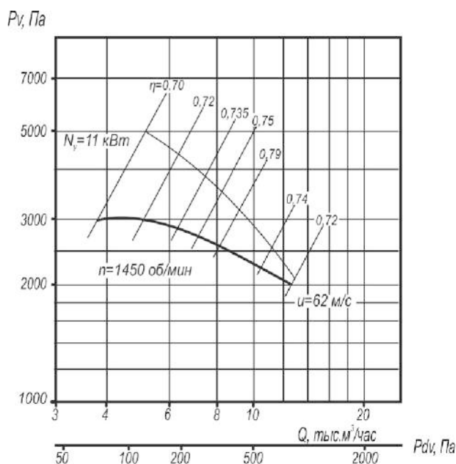
Рис. 21. Аэродинамическая характеристика вентилятора ВЦ 5-35 №8.
