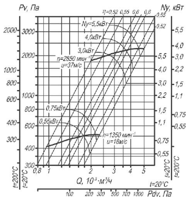
Рис. 11. Аэродинамическая характеристика вентилятора ВЦ 14-46 №2,5.
