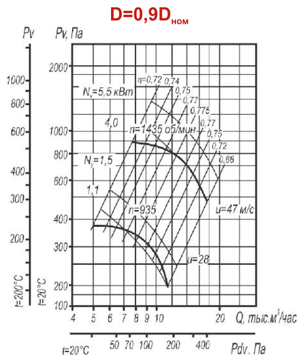
Рис. 57. Аэродинамическая характеристика вентилятора ВР 80-75 №6,3 исп-1; 5 D=0,9D_{\text{НОМ}} .
