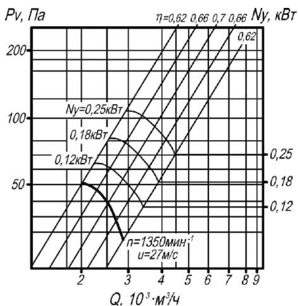
ВО 14-320 №3,15
