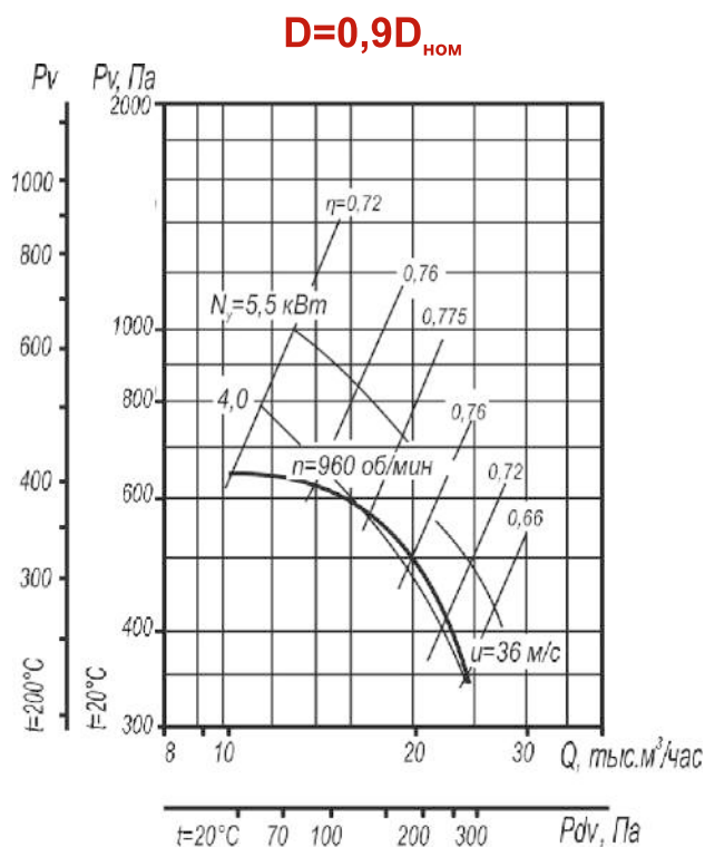
Рис. 62. Аэродинамическая характеристика вентилятора BP 80-75 №8 исп-1; 5, D=0,9D ном .
