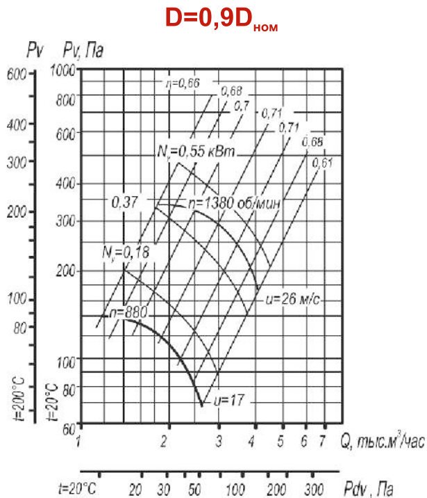
Рис. 47. Аэродинамическая характеристика вентилятора ВР 80-75 №4 исп-1, D=0,9D_{\text{НОМ}} .
