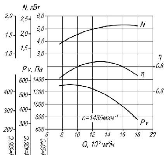
Рис. 219. Аэродинамическая характеристика вентилятора ВР 86-77 №6,3 ДУ.
