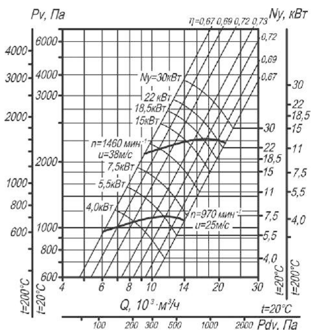
Рис. 14. Аэродинамическая характеристика вентилятора ВЦ 14-46 № 5.
