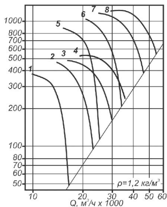
Рис. 183. Аэродинамические характеристики вентилятора ВО 30-160 №9.
