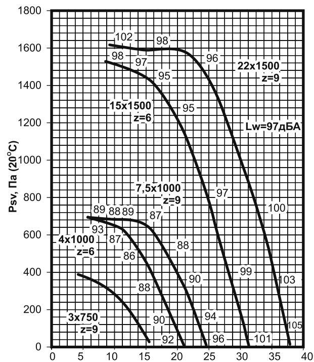
Рис. 151. Аэродинамическая характеристика вентилятора ВКРВм №8.
