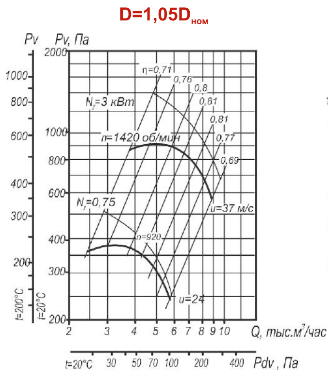
Рис. 54. Аэродинамическая характеристика вентилятора BP 80-75 №5 исп-1; 5 D=1,05D_{\text{НОМ}} .
