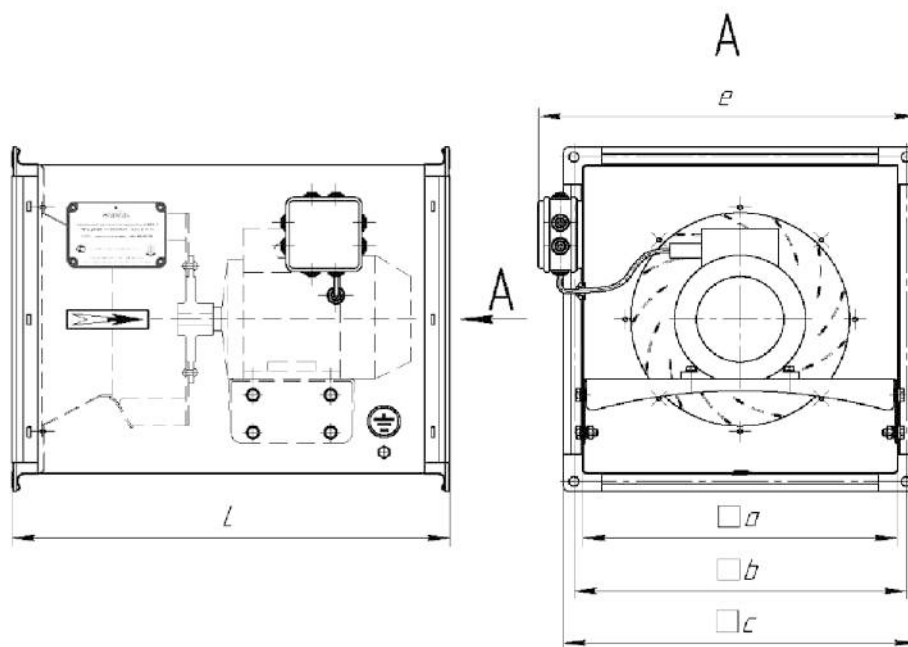
Рис. 191. Габаритные размеры вентиляторов КВК.
