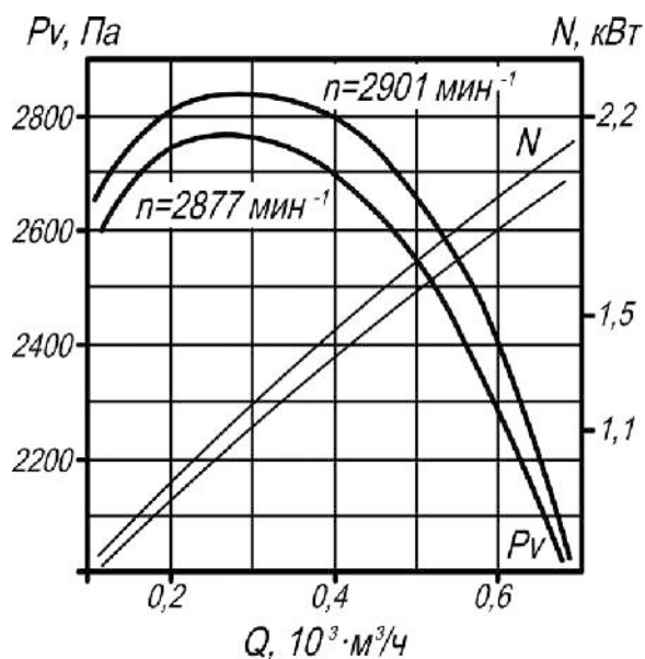
Рис. 87. Аэродинамическая характеристика вентилятора ВР 132-30 №4 исп-1.
