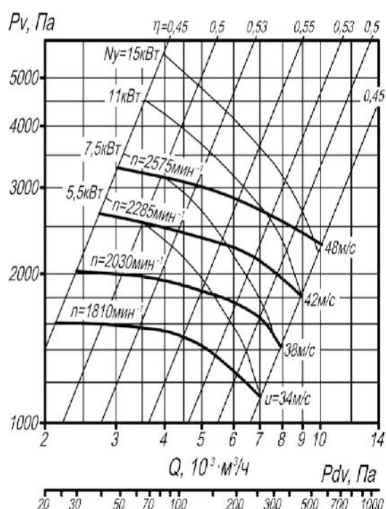
Рис. 114. Аэродинамическая характеристика вентилятора ВР №140-40 №5 исп-1;5.
