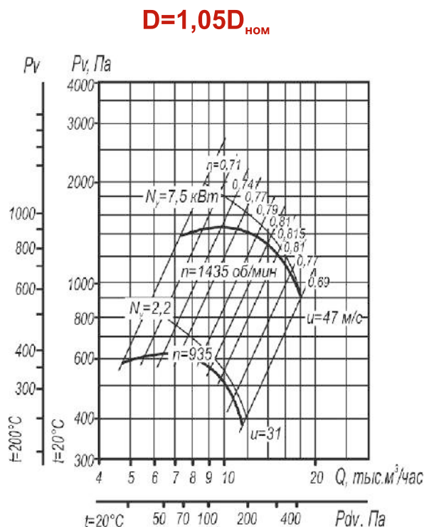
Рис. 59. Аэродинамическая характеристика вентилятора ВР 80-75 №6,3 исп-1; 5 D=1,05D_{\text{НОМ}} .
