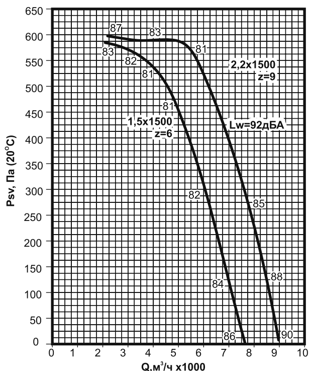
Рис. 147. Аэродинамическая характеристика вентилятора ВКРВм №5.
