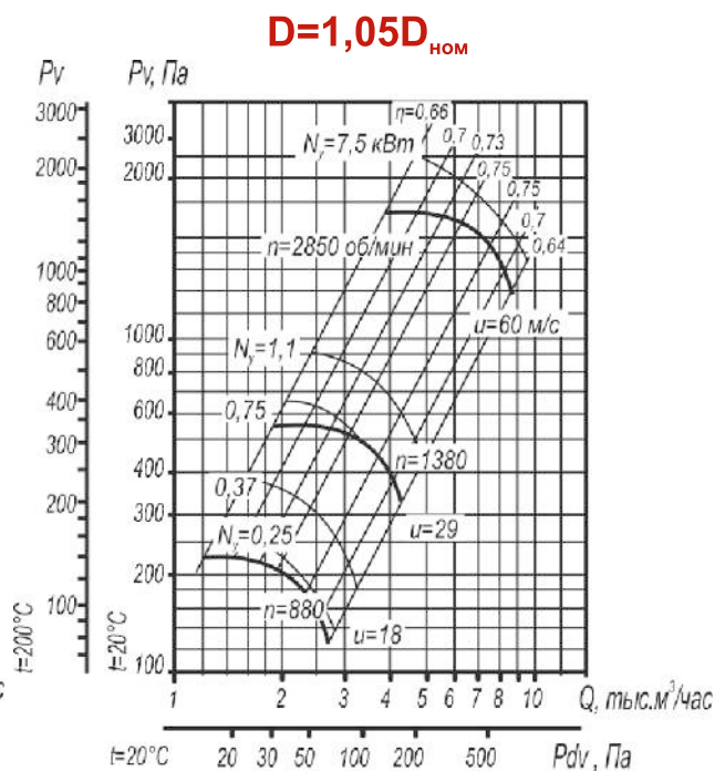
Рис. 49. Аэродинамическая характеристика вентилятора ВР 80-75 №4 исп-1, D=1,05D_{\text{ном}} .
