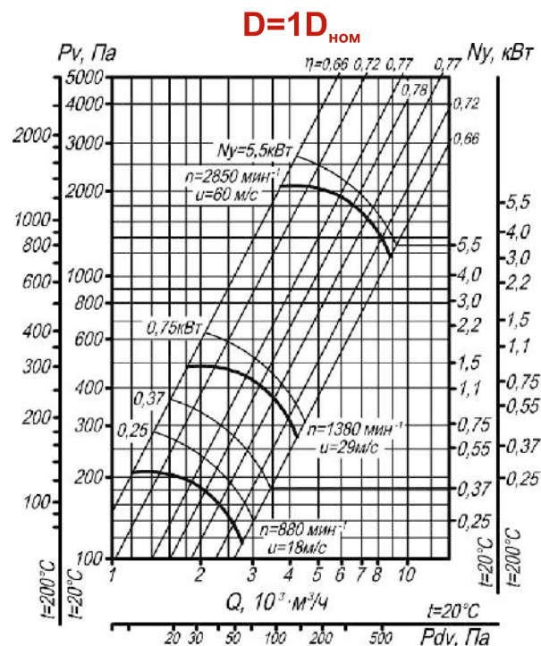
Рис. 46. Аэродинамическая характеристика вентилятора ВР 80-75 №4 исп-1, D=1D_{\text{НОМ}} .
