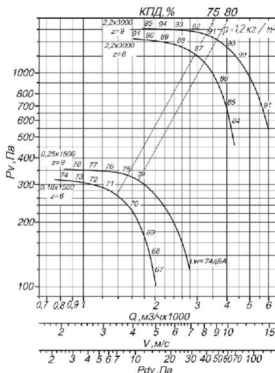
Рис. 76. Аэродинамическая характеристика вентилятора BP 80-75 №3,55 исп-1.
