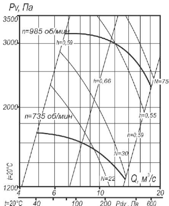
Рис. 118. Аэродинамическая характеристика вентилятора BP №140-40 №12,5.
