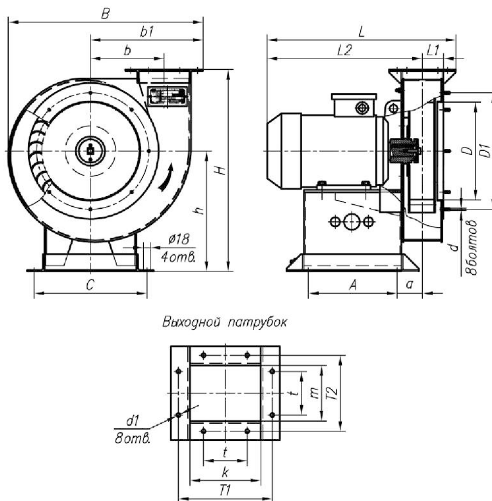
Рис. 97. Габаритные и присоединительные размеры вентиляторов ВР 12-26 (углерод. сталь).
