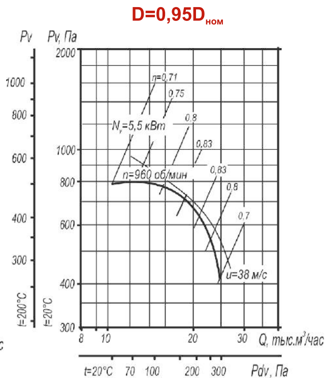
Рис. 63. Аэродинамическая характеристика вентилятора BP 80-75 №8 исп-1; 5 D=0,95D ном .
