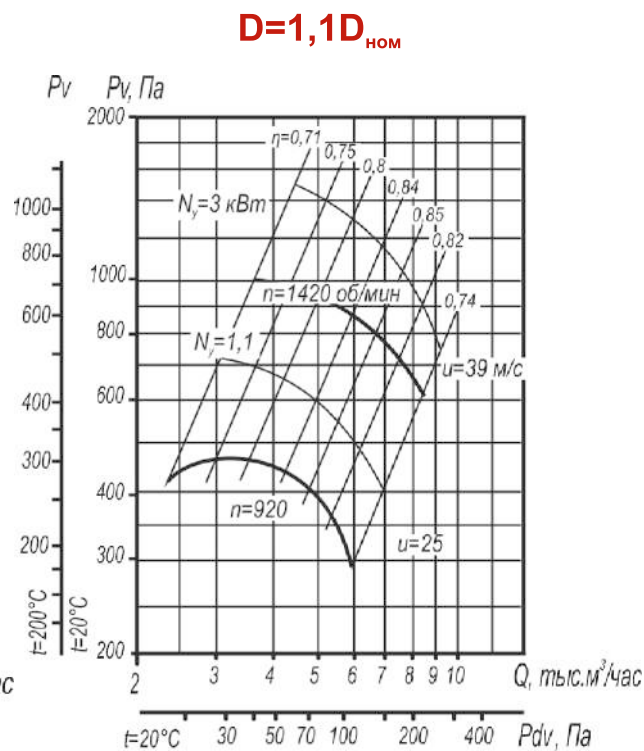
Рис. 55. Аэродинамическая характеристика вентилятора BP 80-75 №5 исп-1; 5 D=1,1D_{\text{НОМ}} .
