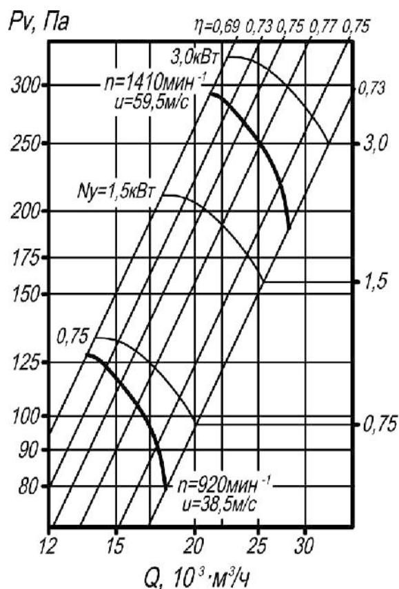
Рис. 170 Аэродинамические характеристики вентиляторов осевых ВО 14-320 №5; №6,3; №8; №10.
