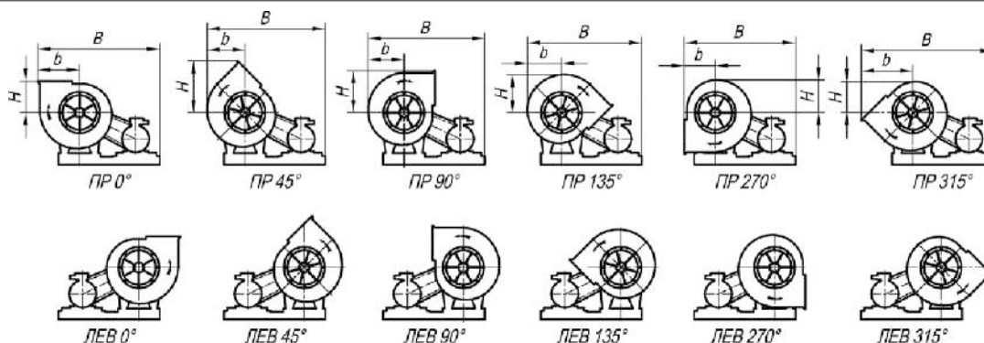
Рис. 26. Положения корпуса вентилятора ВР 9-55 исп-5.
