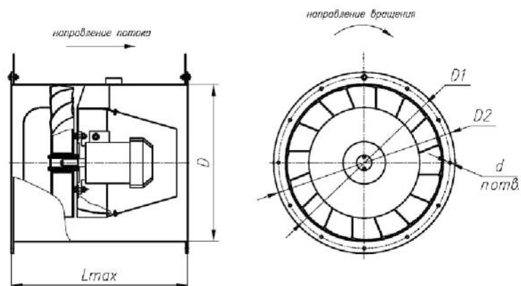
Компоновка 2
