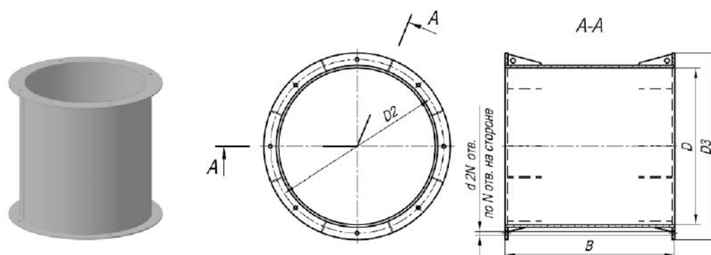
Рис. 156. Габаритные и присоединительные размеры стаканов для крышных вентиляторов.
