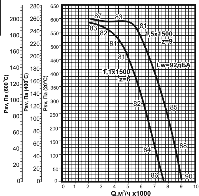
Рис. 249. Аэродинамическая характеристика вентилятора ВКРВм №5 ДУ
