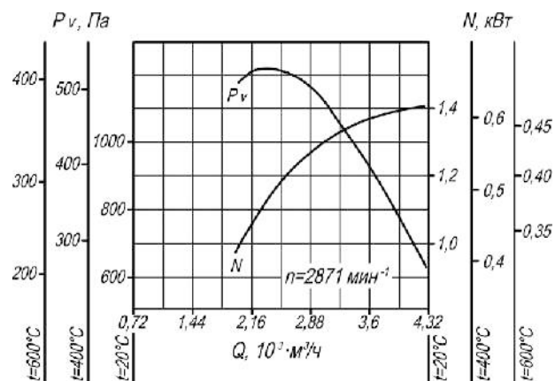
Рис. 216. Аэродинамическая характеристика вентилятора ВР 86-77 №3,15 ДУ.
