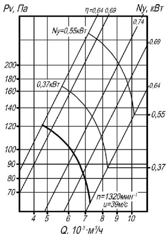
ВО 14-320 №8
