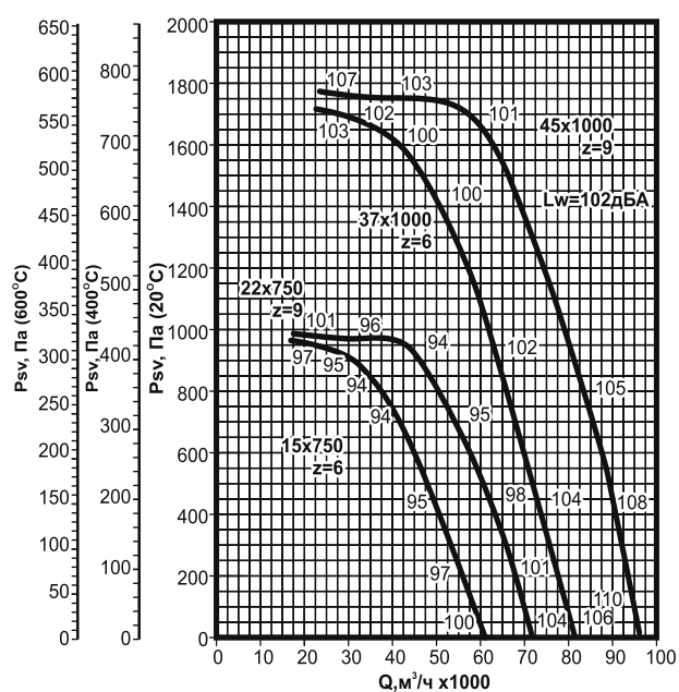
Рис. 257. Аэродинамическая характеристика вентилятора ВКРВм №12,5 ДУ.
