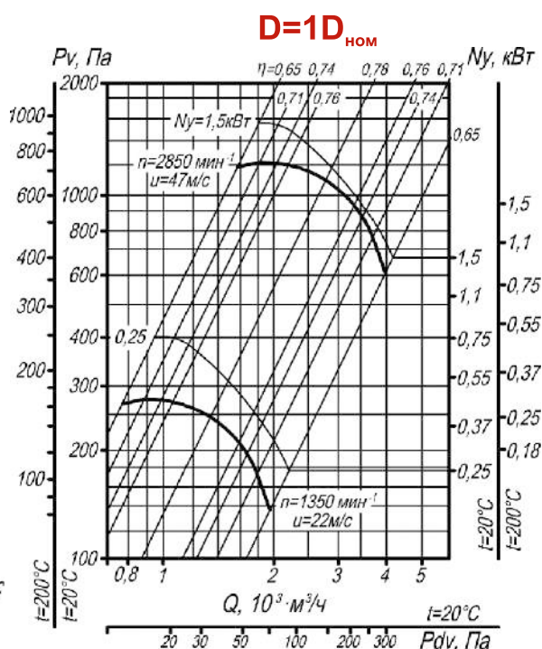
Рис. 41. Аэродинамическая характеристика вентилятора ВР 80-75 №3,15 исп-1, D=1Dном.
