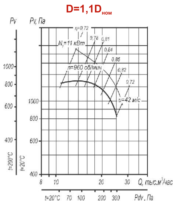
Рис. 65. Аэродинамическая характеристика вентилятора ВР 80-75 №8 исп-1; 5 D=1,1D_{\text{ном}} .
