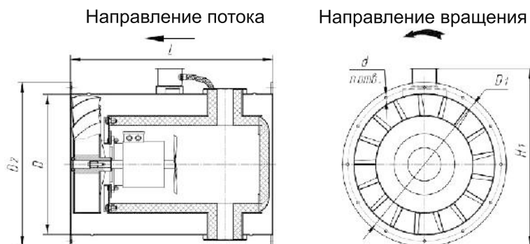
Компоновка 3
