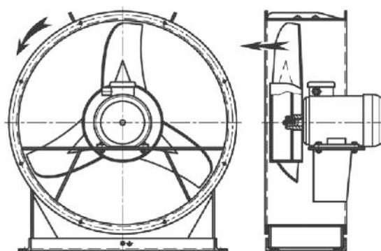
Исполнение 2
