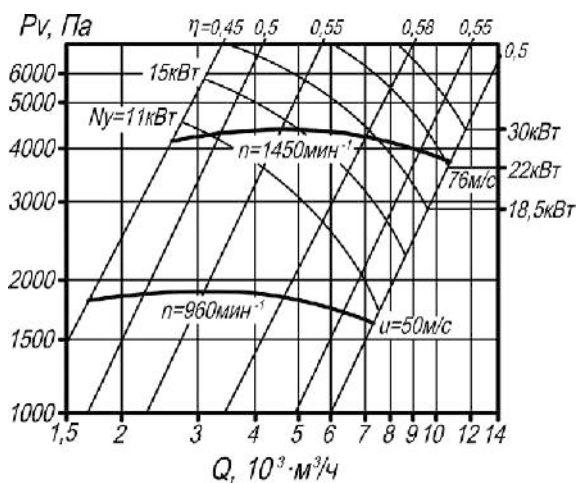
Рис. 92. Аэродинамическая характеристика вентилятора ВР 132-30 №9 исп-1.
