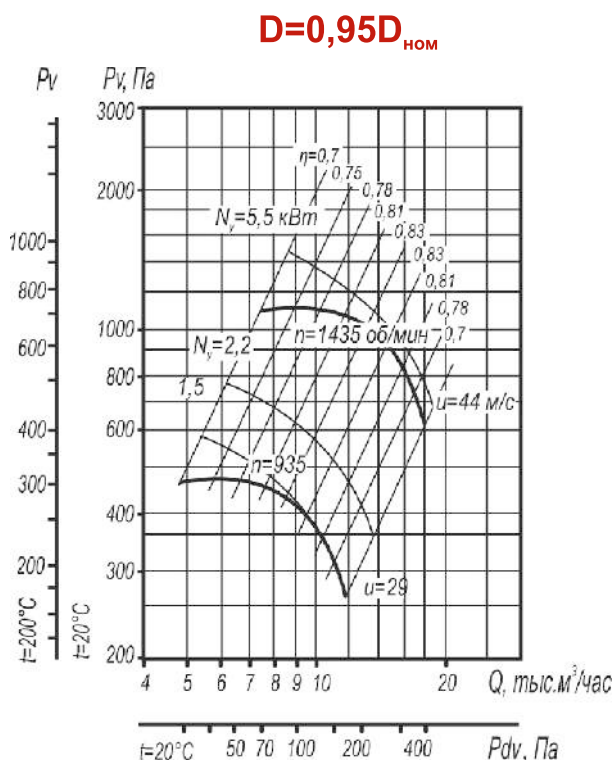
Рис. 58. Аэродинамическая характеристика вентилятора ВР 80-75 №6,3 исп-1; 5, D=0,95D_{\text{НОМ}} .
