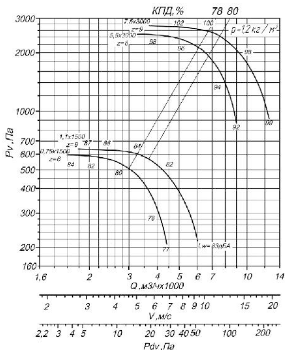
Рис. 77. Аэродинамическая характеристика вентилятора BP 80-75 №4,5 исп-1.
