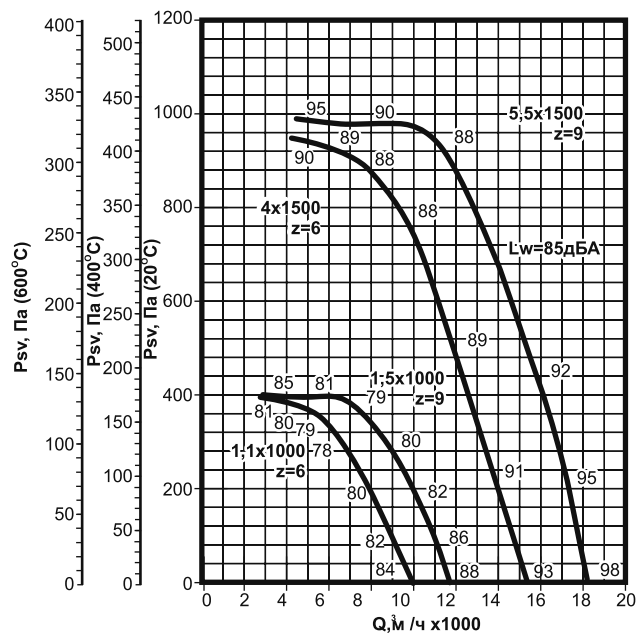
Рис. 251. Аэродинамическая характеристика вентилятора ВКРВм №6,3 ДУ.
