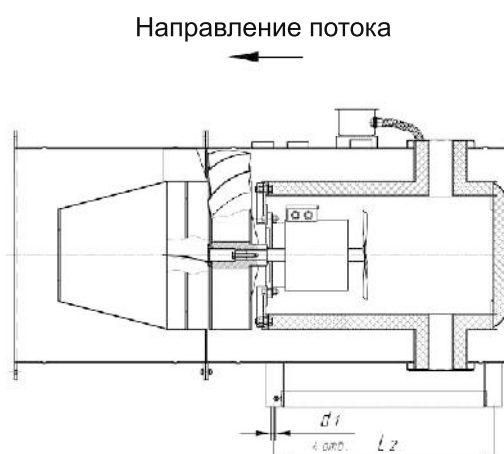
Рис. 261. Габаритные и присоединительные размеры осевых вентиляторов дымоудаления ВОДм-ДУ.
