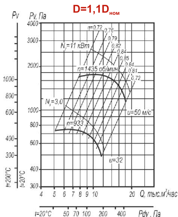
Рис. 60. Аэродинамическая характеристика вентилятора BP 80-75 №6,3 исп-1; 5 D=1,1D ном .
