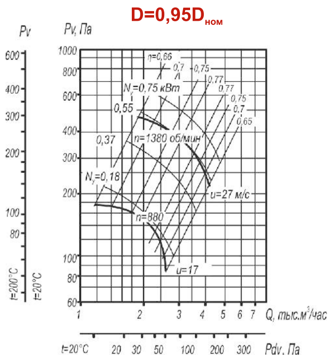
Рис. 48. Аэродинамическая характеристика вентилятора ВР 80-75 №4 исп-1, D=0,95D_{\text{ном}} .
