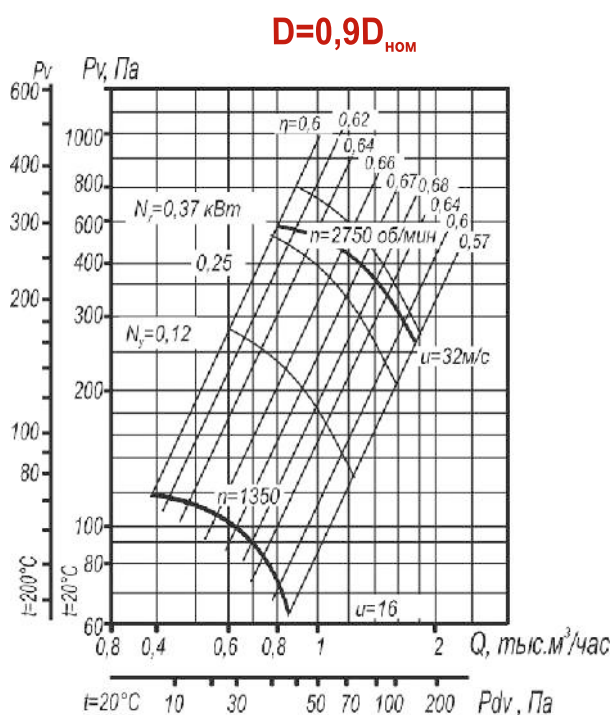
Рис. 37. Аэродинамическая характеристика вентилятора ВР 80-75 №2,5 исп-1, D=0,9D НОМ .
