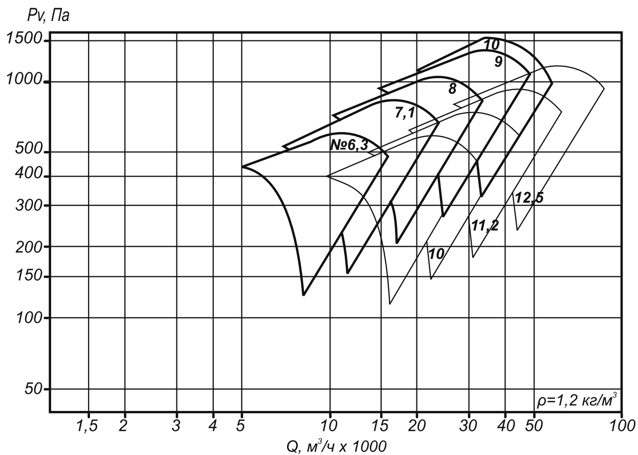
Рис. 187. Область аэродинамических параметров ВО 30-160.
