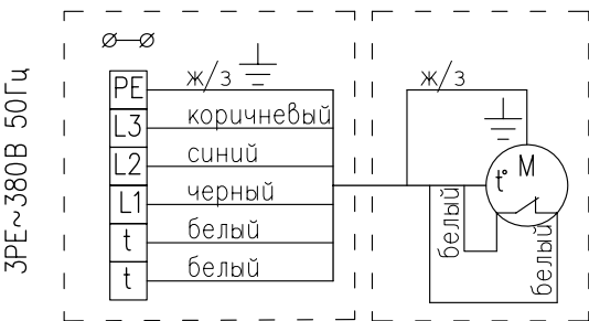
Схема В. Подключение к сети 380 В 50 Гц
