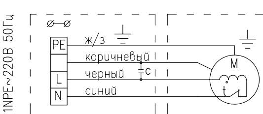
Схема Б. Подключение к сети 220 В 50 Гц
