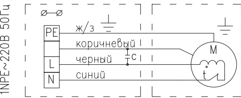
Схема Б. Подключение к сети 220 В 50 Гц
