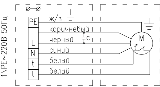
Схема А. Подключение к сети 220 В 50 Гц
