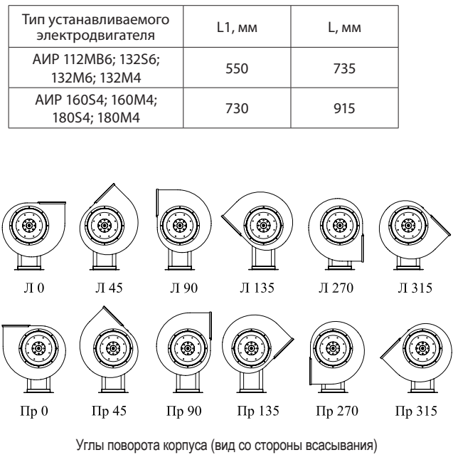
Углы поворота корпуса (вид со стороны всасывания)
