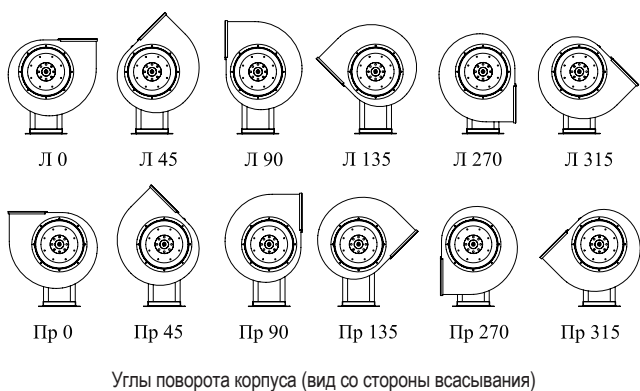
Углы поворота корпуса (вид со стороны всасывания)
