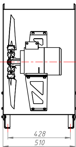
80/90/100 габарит ЭД
