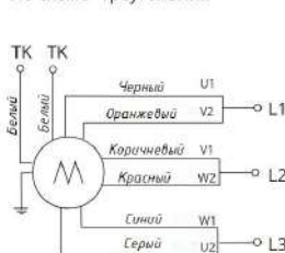
По схеме "треугольник"
