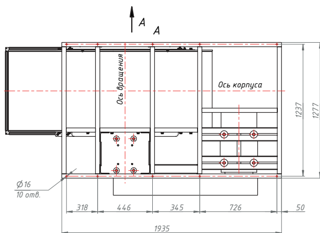
ВЫХОДНОЙ ФЛАНЕЦ
