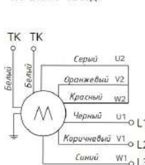
По схеме "звезда"
