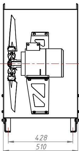
90/100 габарит ЭД
