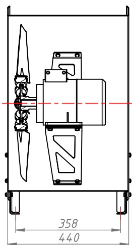
71 габарит ЭД
