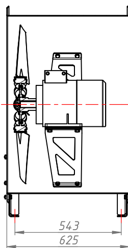
112/132 габарит ЭД
