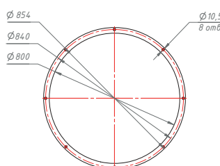
ВХОДНОЙ ФЛАНЕЦ
