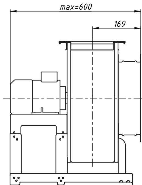
ВХОДНОЙ ФЛАНЕЦ
