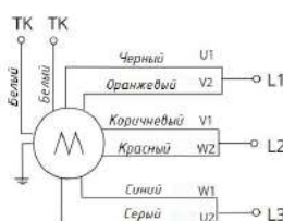
По схеме "треугольник"
