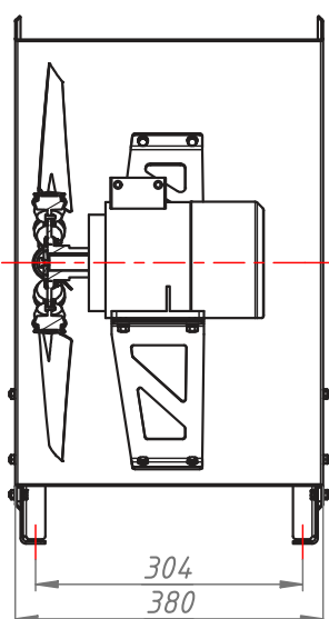
63 габарит ЭД
