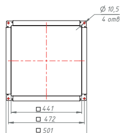
ВЫХОДНОЙ ФЛАНЕЦ
