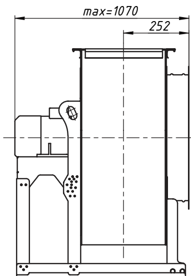
ВХОДНОЙ ФЛАНЕЦ
