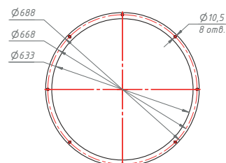
ВЫХОДНОЙ ФЛАНЕЦ
