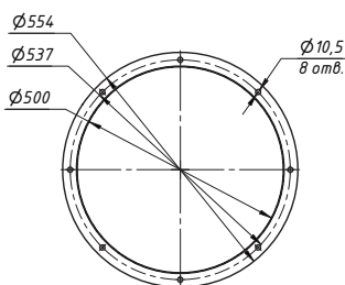
ВЫХОДНОЙ ФЛАНЕЦ
