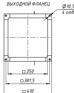
ВЫХОДНОЙ ФЛАНЕЦ
