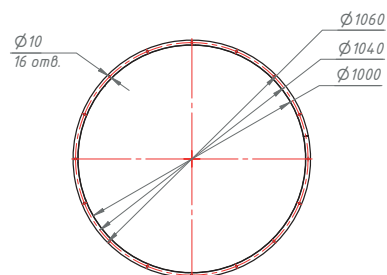
ВЫХОДНОЙ ФЛАНЕЦ
