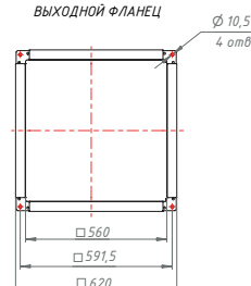
ВЫХОДНОЙ ФЛАНЕЦ
