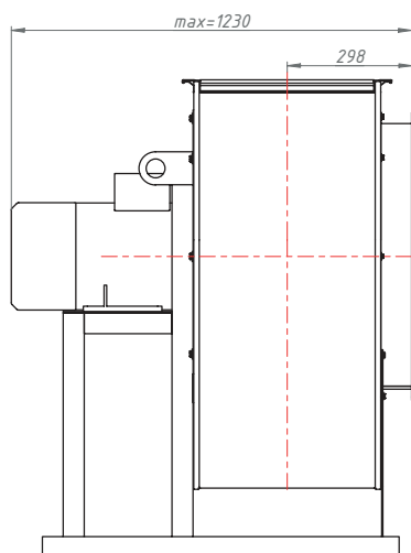
ВХОДНОЙ ФЛАНЕЦ
