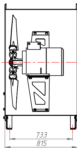
160/180 габарит ЭД
