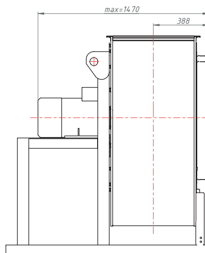
ВХОДНОЙ ФЛАНЕЦ
