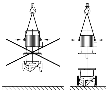
Рис. 4: Транспортировка двигателя
