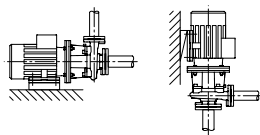
Рис. 38: Вид BL
