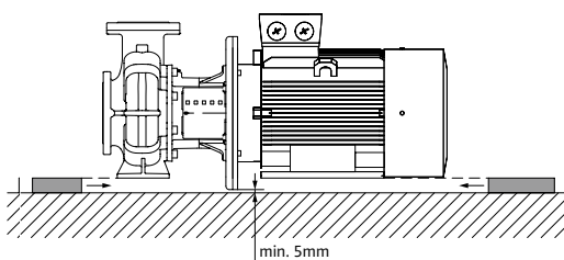
Рис. 42: Примеры монтажа BL
