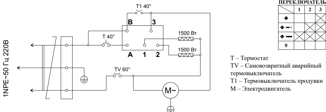
Рисунок 4. Электрическая схема тепловентилятора КЭВ-3С31Е
