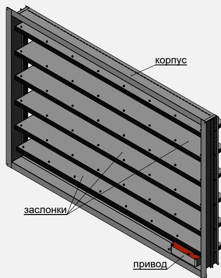
Сигмавент-60-НО(СЛ)-АхВх150-SVF(24)
