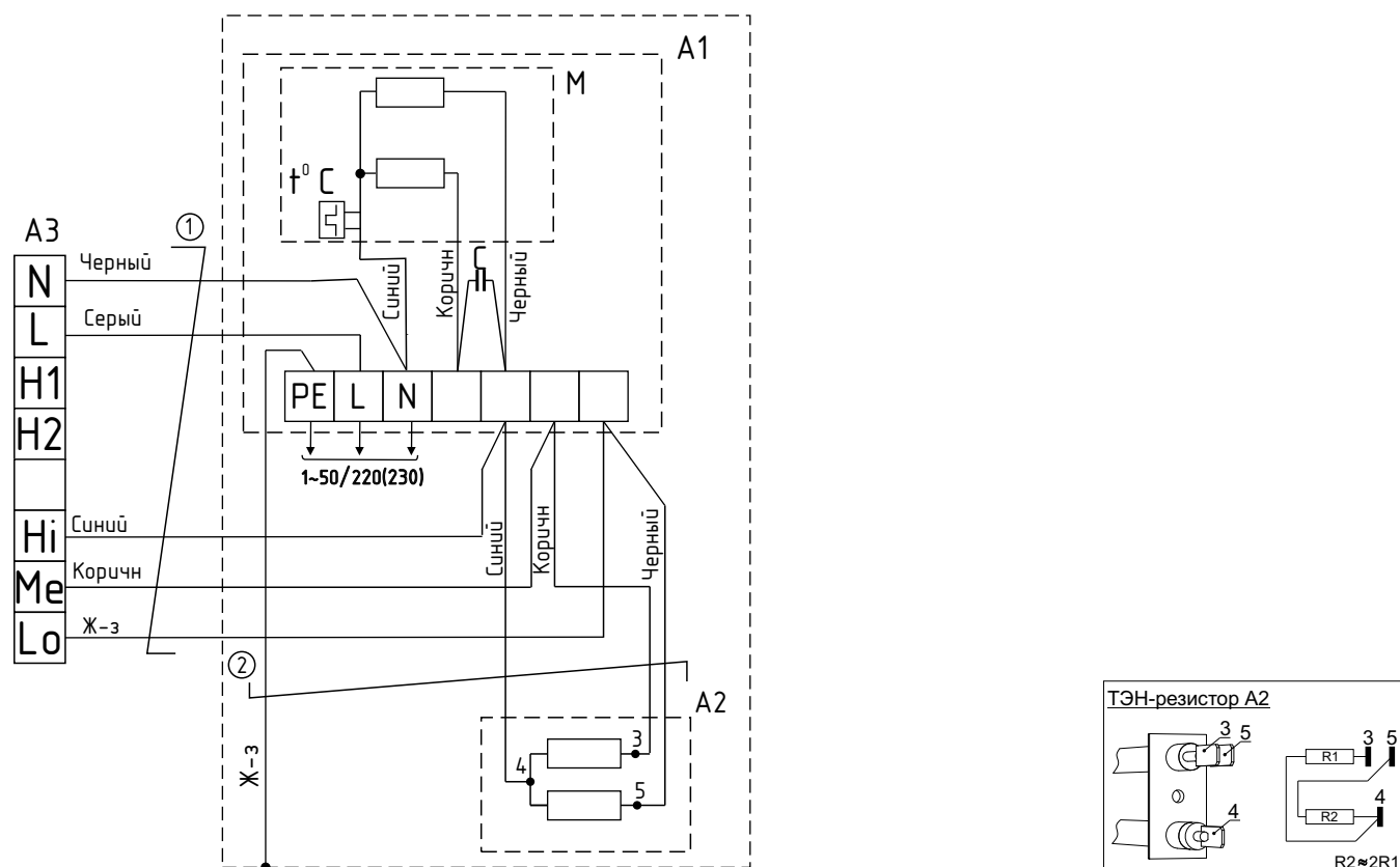
Рисунок 7. Электрическая схема дестратификаторов ВО-4 (КЭВ-Д4-1), ВО-4 (КЭВ-Д4-2), ВО-4,5 (КЭВ-Д4,5-2)
