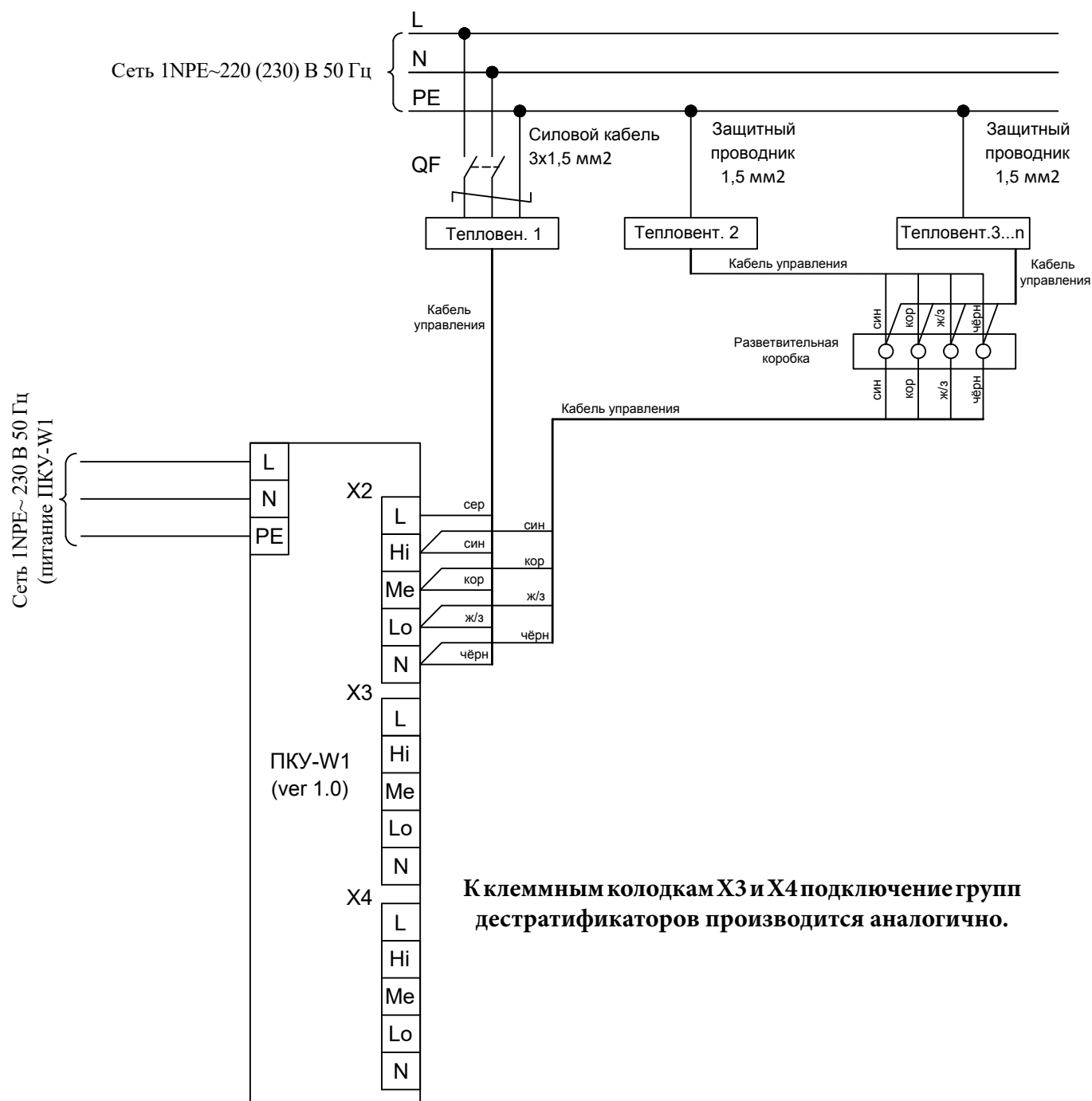
Рисунок 4. Схема подключения одной группы дестратификаторов к ПКУ-W
